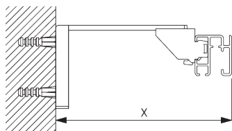
Smart Fix SG 11200 - SG 11205 en steun SG 3603:
