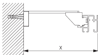
Square Smart Fix SG 11210 - SG 11215 en steun SG 3603:
