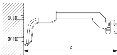
Universal Smart Fix SG 11154 - SG 11156 en steun SG 3603:
