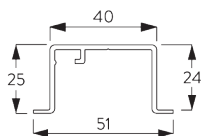
SG 10862 Inbouwprofiel
