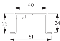
SG 10862 Inbouwprofiel
