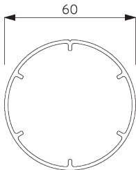
SG 11037 Profiel
