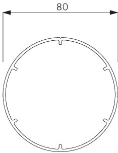
SG 11003 Profiel
