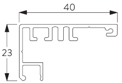
SG 11418 Zijgeleidingsprofiel
