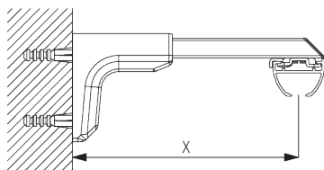
Universal Smart Fix SG 11154 - SG 11156 en spanner SG 3825: Schröef SG 11158 (M4x12) nodig.
