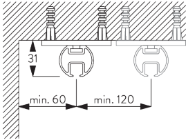
Steun SG 6124
