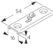
SG 6124 Steun
