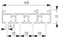
SG 10124 Profil 4 canaux
