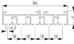
SG 10125 Profil 5 canaux
