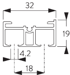
SG 10122 Profil 2 canaux
