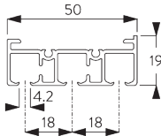
SG 10123 Profil 3 canaux
