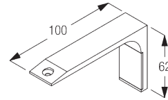
SG 11669 Afstandssteun
