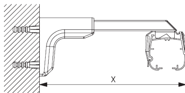
Universal Smart Fix SG 11154 - SG 11156 en steun SG 2302: Schroef SG 10492 (M4x8) nodig.
