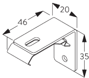
SG 2343 Wandsteun 46 mm
