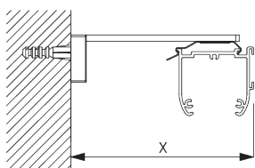
Square Smart Fix SG 11210 - SG 11215 en steun SG 2616: Schroef SG 10395 (M4x6) nodig.
