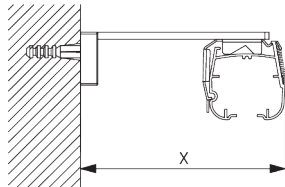
Square Smart Fix SG 11210 - SG 11215 en steun SG 2302: Schroef SG 10395 (M4x6) nodig.
