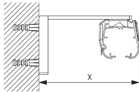
Smart Fix SG 11200 - SG 11205 en steun SG 2302: Schroef SG 10395 (M4x6) nodig.
