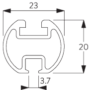
SG 1003p Profil rond
