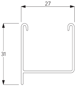
SG 8102 Profiel
