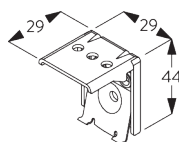
SG 8302 Steun
