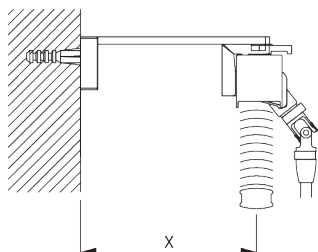
Square Smart Fix SG 11210 - SG 11211 et support SG 10101: Vis SG 10395 (M4x6) nécessaire.
