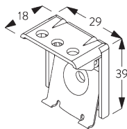
SG 8201 Steun
