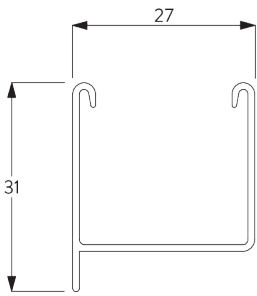
SG 8102 Profiel
