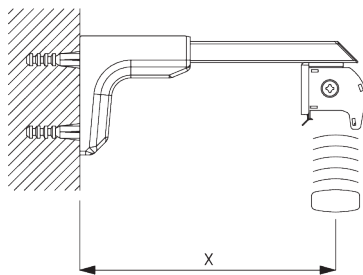
Universal Smart Fix SG 11154 - SG 11156 en steun SG 8302: Schroef SG 10407 (M4x10) nodig.
