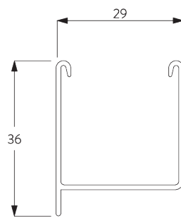
SG 8301 Profiel
