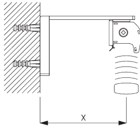
Smart Fix SG 11200 - SG 11201 en steun SG 8302: Schroef SG 10395 (M4x6) nodig.
