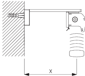
Square Smart Fix SG 11210 - SG 11211 en steun SG 8302: Schroef SG 10395 (M4x6) nodig.
