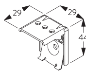
SG 8302 Steun
